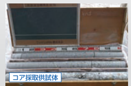
コア採取供試体
